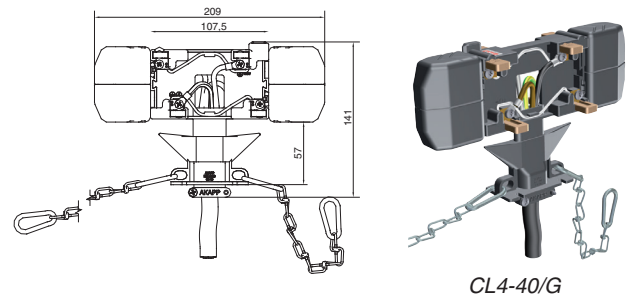
CL4-40/G
