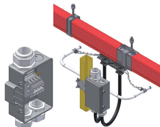
BMV70 + TTB70-4
