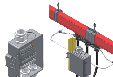
BMV100 + TTB100-7
